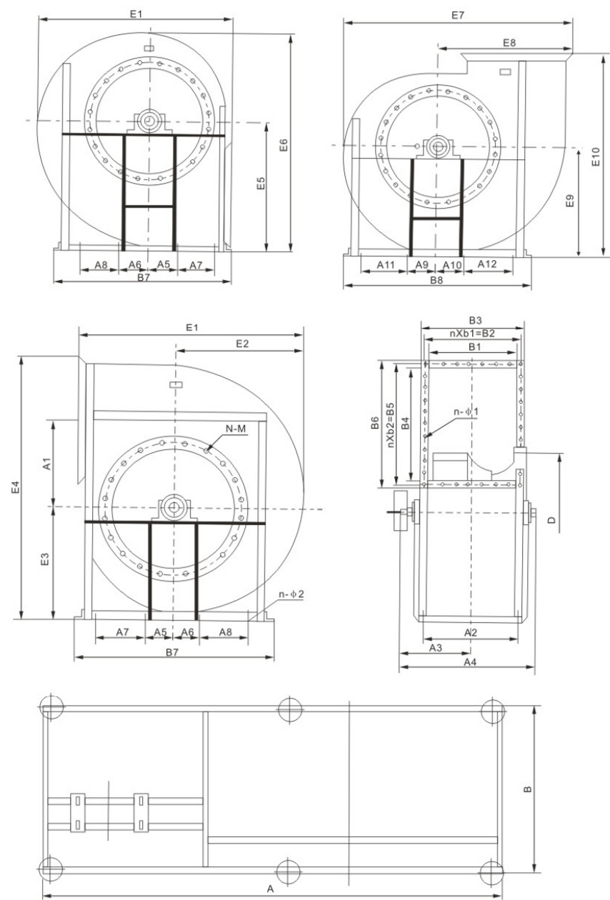
(三)、4-72、4-79系列14E~16E离心风机外形图
