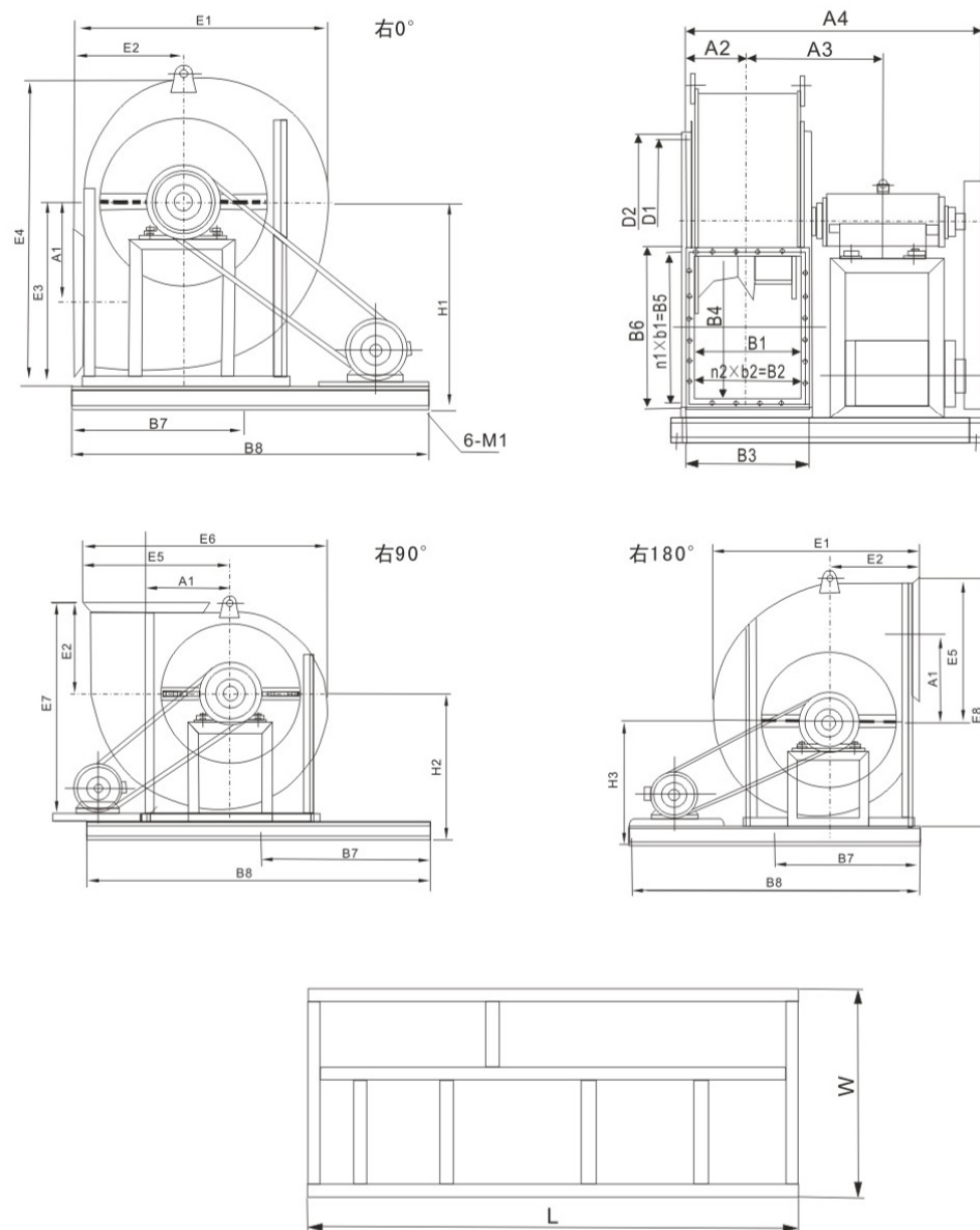
(二)、4-72、4-79系列6C~12C离心风机外形图
